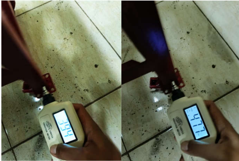
Pengukuran Amplitudo pada Titik Suspensi Kiri
