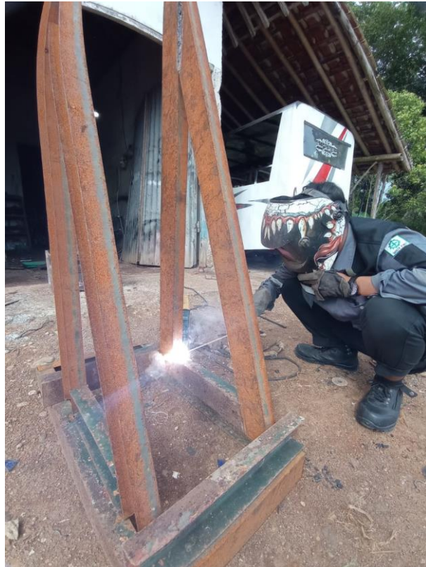
Proses pengelasan pada bagian bawah rangka
