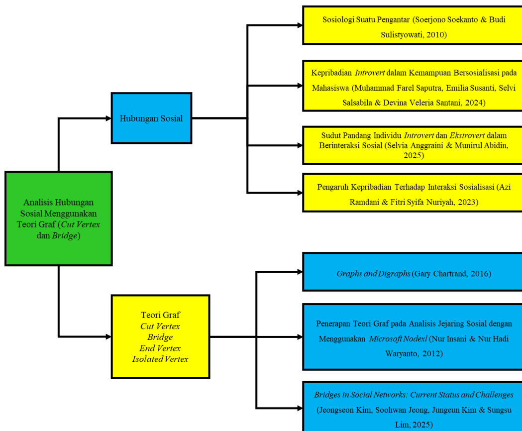
Gambar 1. Mind Map.
